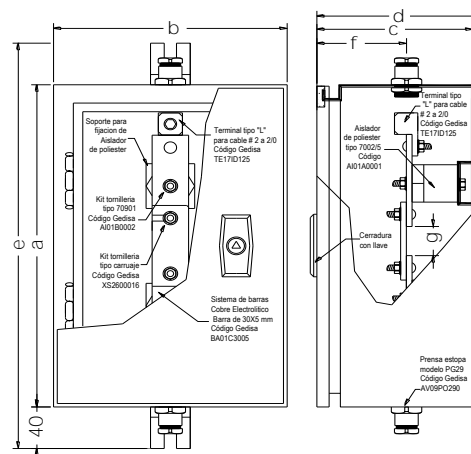
CAJA PARA MEDICION DE TIERRA
