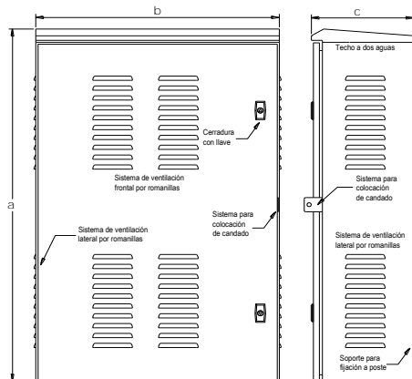
GABINETE PARA TORRES DE ALUMBRADO
