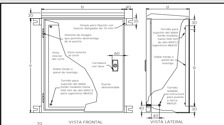
GABINETE TIW NEMA 3R
