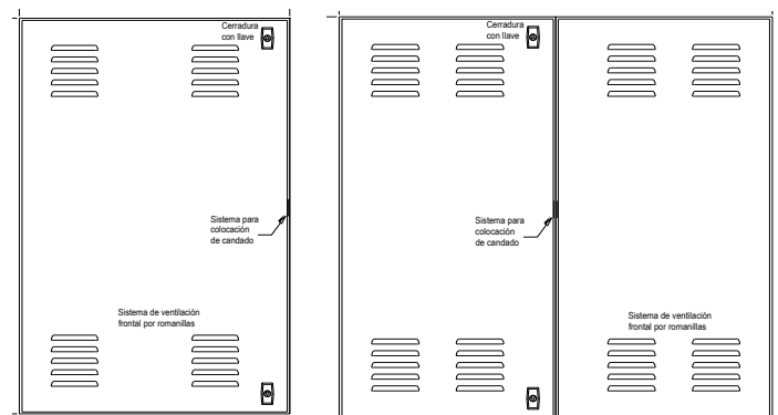
GABINETE METALICO TELEFONICO
