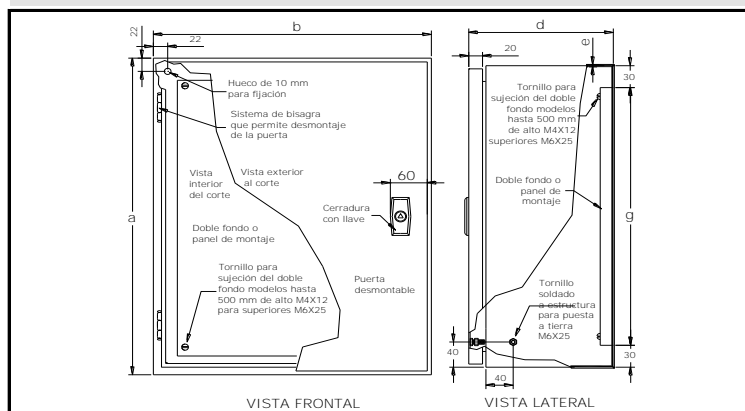
GABINETE TI NEMA 1
