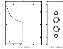
CAJA DE PASO NEMA 1
