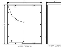
CAJA DE PASO NEMA 4
