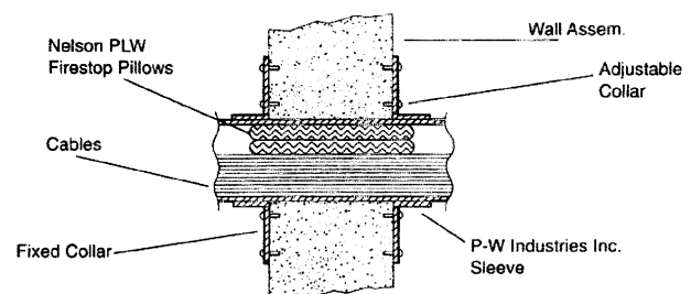
Barrera contra fuego Figura artículo 318-3(a)(2)
