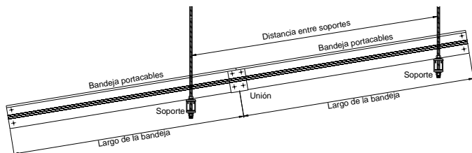
Localización de soportes en secciones rectas inclinadas Figura 5
