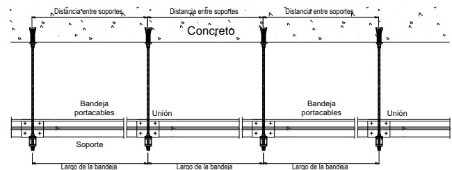
Localización no recomendada de soportes en secciones rectas Figura 4
