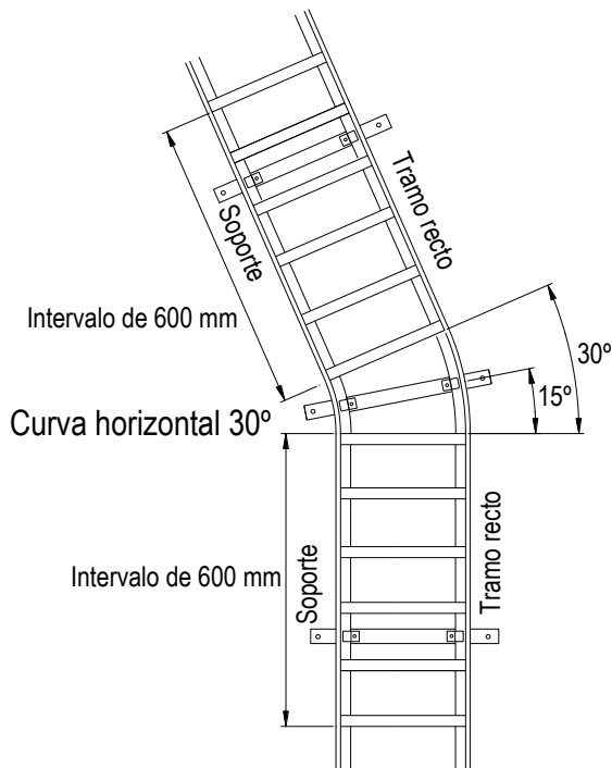
Soportes en curva horizontal a 30° Figura 9
