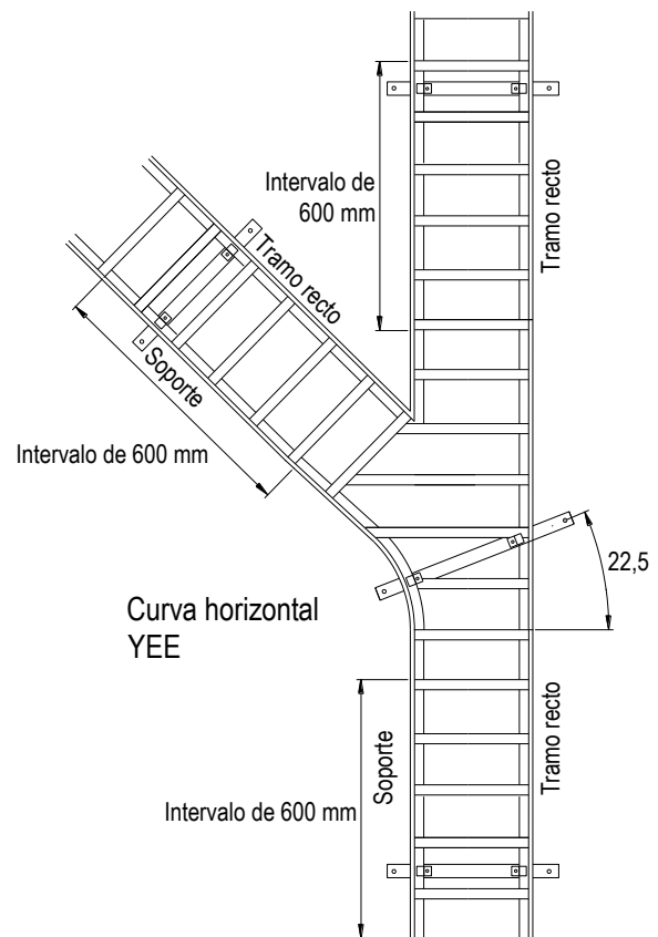
Soportes en curva horizontal YEE Figura 10
