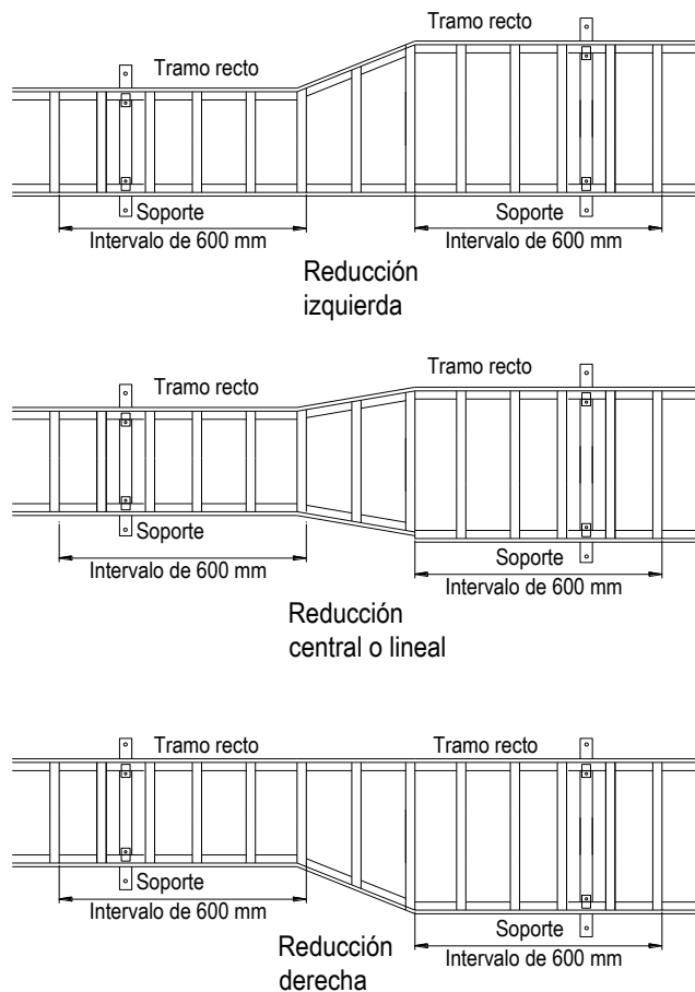
Soportes en reducciones Figura 11
