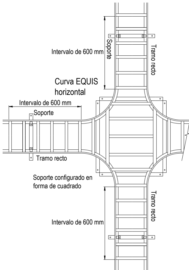
Soportes en Curva horizontal tipo Equis Figura 15
