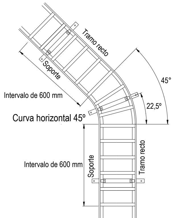
Soportes en curva horizontal a 45° Figura 8
