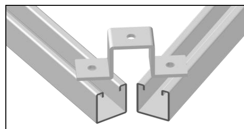
Detalle de arreglo de soporteria Figura 12
