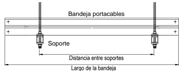
Instalación de bandejas portacables Figura 1
