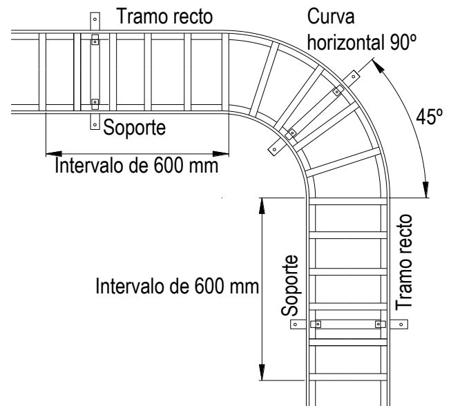
Soportes en curva horizontal 90° Figura 6
