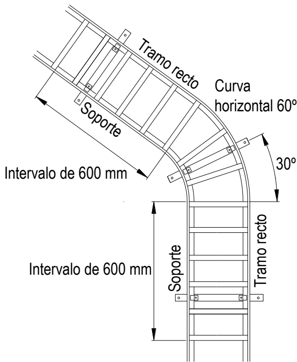
Soportes en curva horizontal a 60° Figura 7
